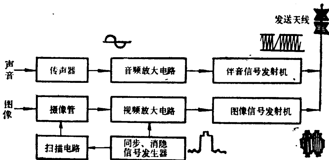
图1-1 电视信号的发送
