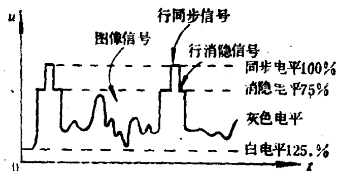
图1-6 图象信号
