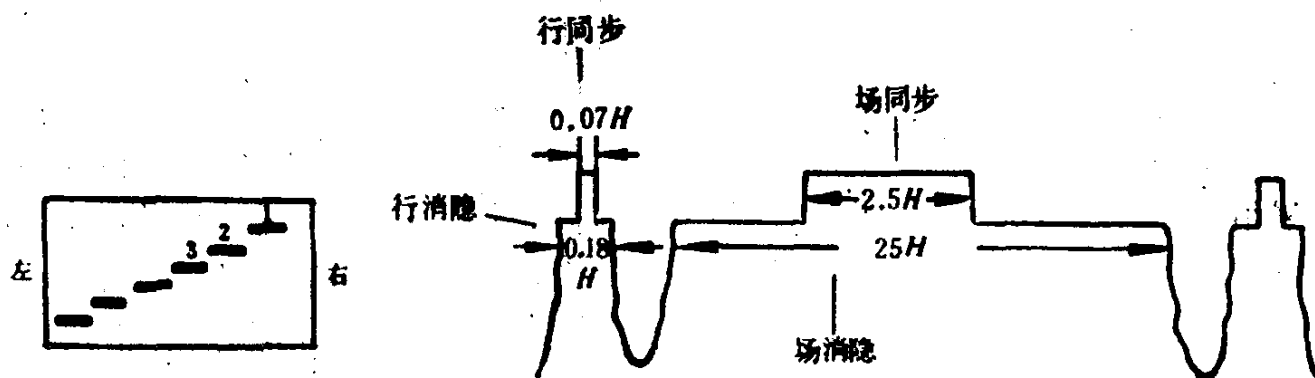
图1-7 行扫描周期偏大时的图象
