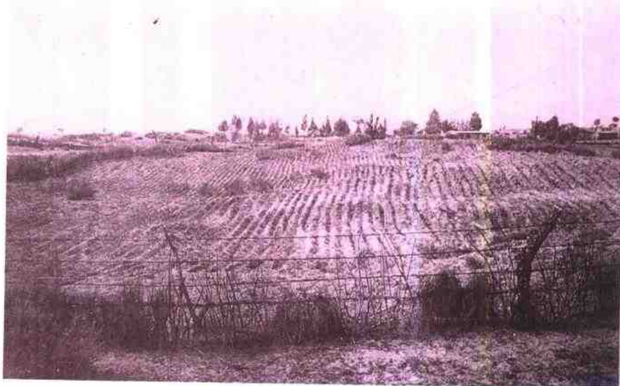
照片1 库伦旗茫汉苏木海斯嘎查耕地沙漠化情景
