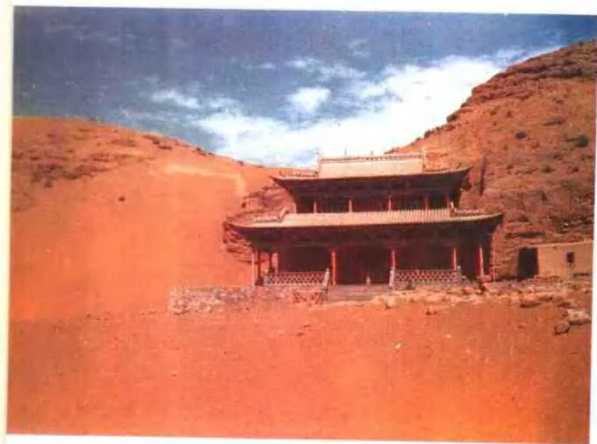
照片 27 石空山已被流沙湮埋
