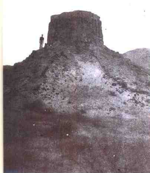
照片 18 科尔沁草原之风蚀残丘,黑土之下 即为白沙 摄于敖汉旗康家营子乡庙下村
