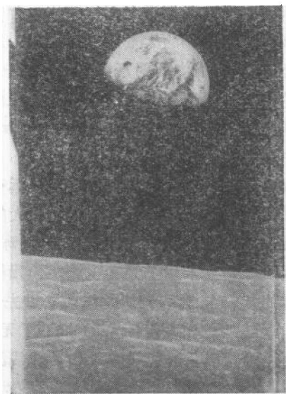
图 0.1 在月球上拍摄的地球的照片
