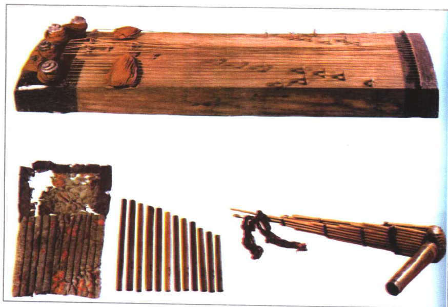
木瑟长116厘米，四个弦钮二十五弦及弦柱都很完整。竽，长为90厘米二十二管分列前后两排。十二音律管，一套12支，发现时插在绣花袋内。
