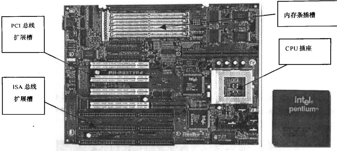
图 1.1.2 主机板示意图
