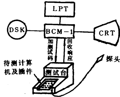
图1.1-6 自动测试仪
