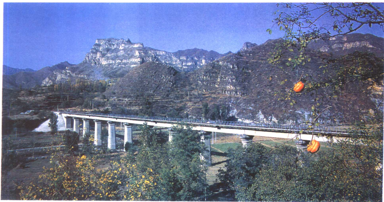
北京矿务局工程公司 1966 年建设的陈磁铁路辛庄大桥
