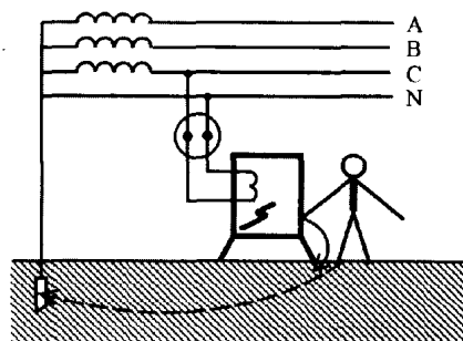
图 1.1 单极接触触电示意图
