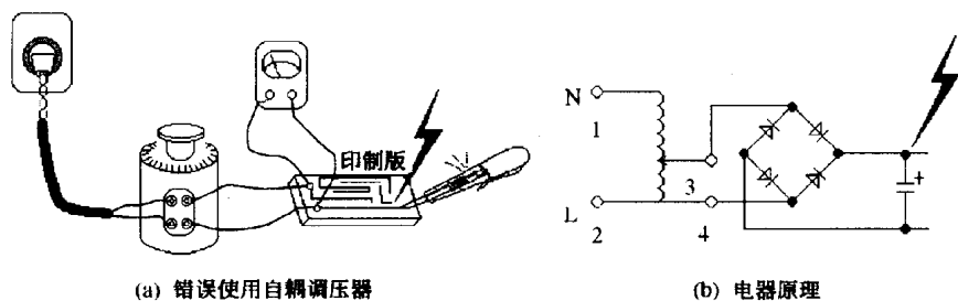
图 1.3 错误使用自耦调压器
