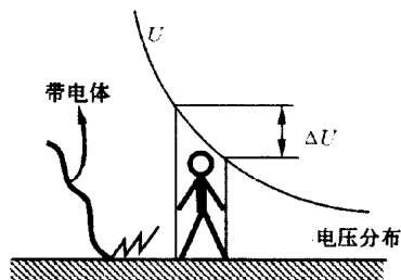
图 1.5 跨步电压使人触电
