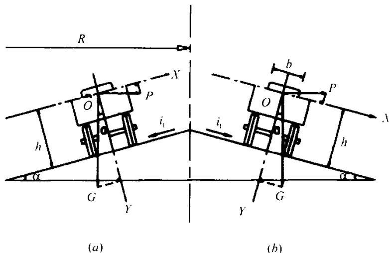
图 2-1 汽车在曲线上行驶的横向力 (a)内侧;(b)外侧
