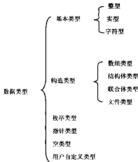
图2-1 C语言数据类型
