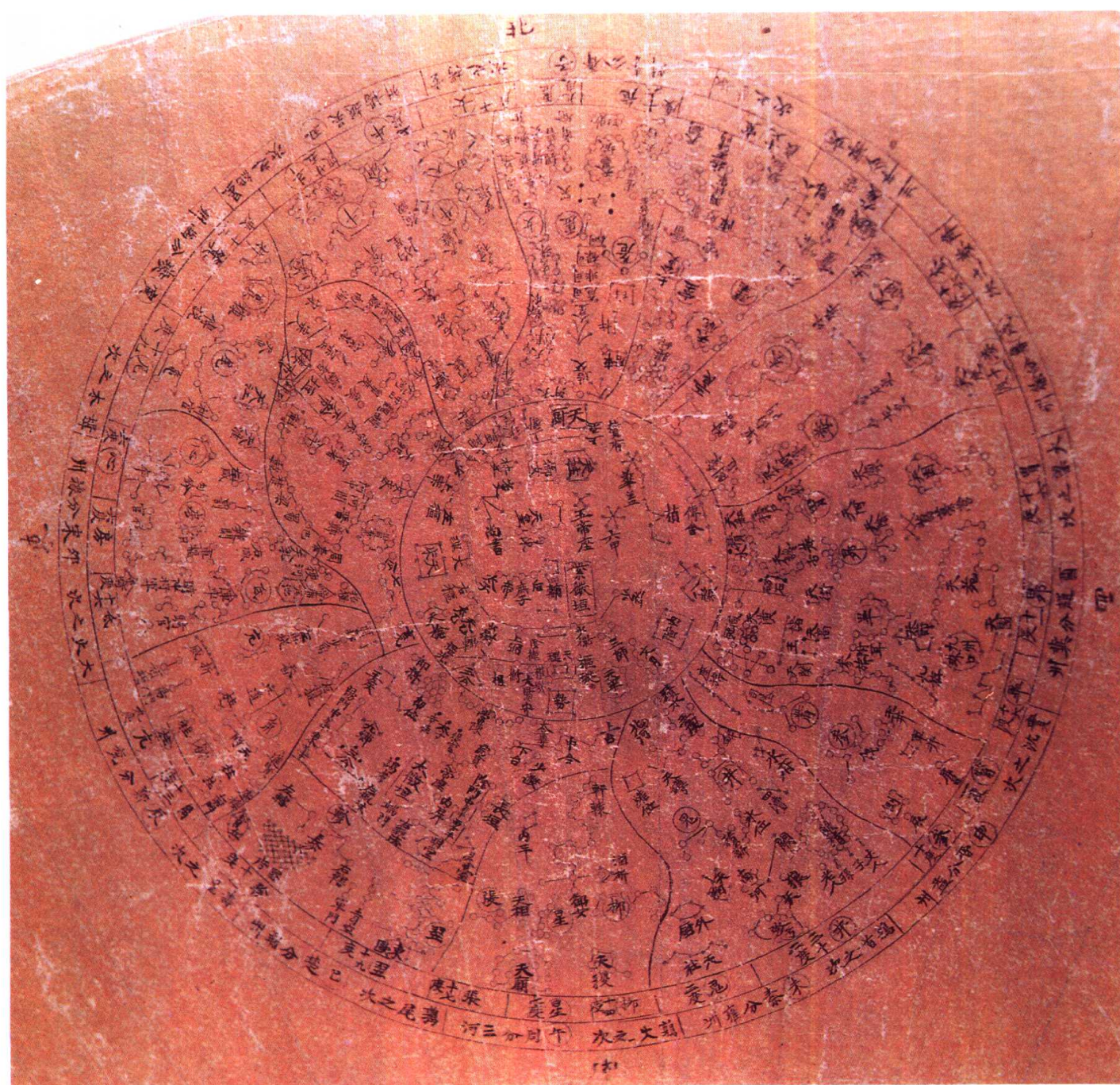
彩图版 9—2 南京博物院藏明代扇面星图
