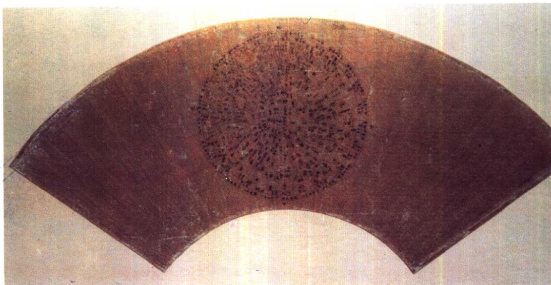
彩图版 9—1 南京博物院藏明代扇面星图(全貌),绘于明嘉靖或万历年间
