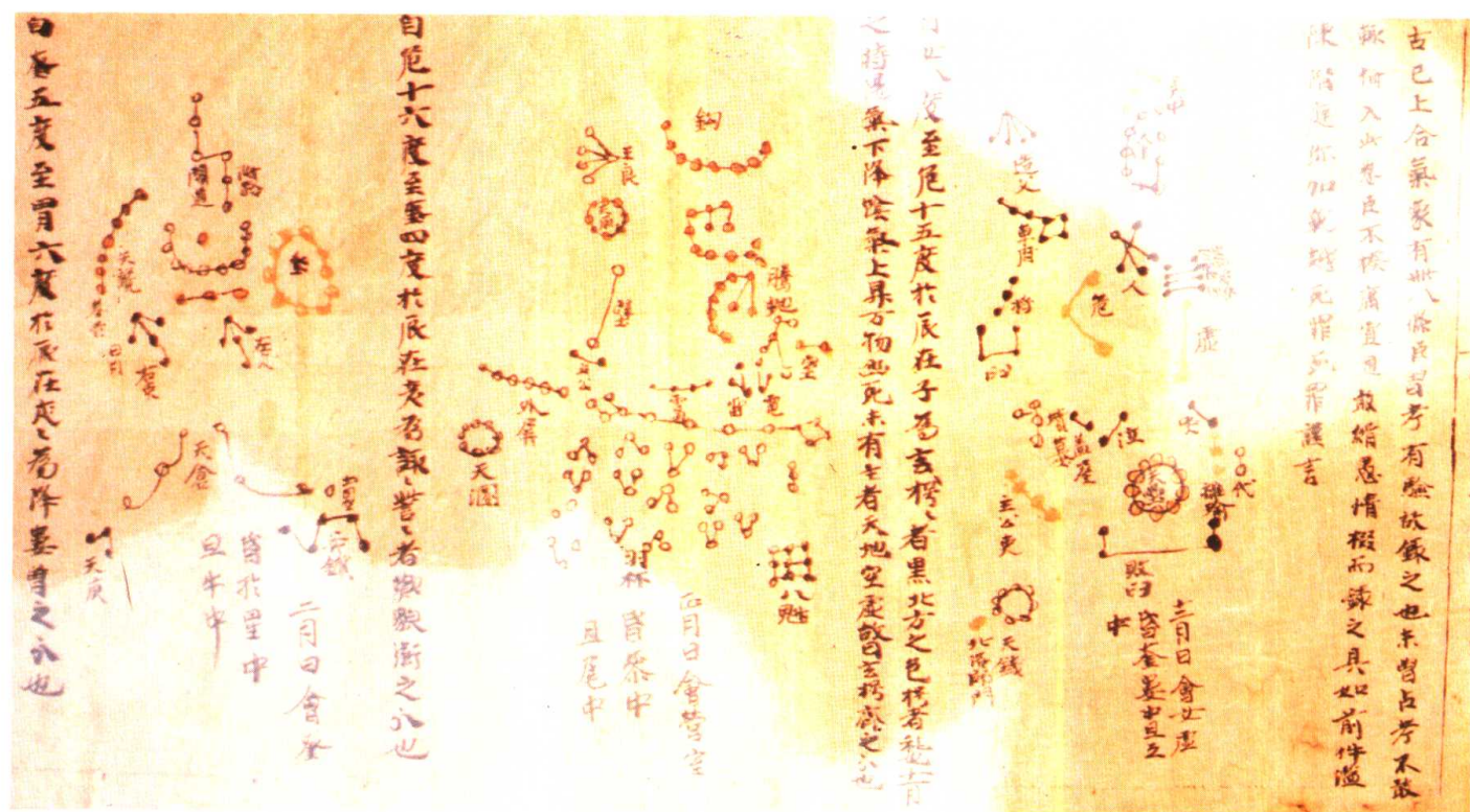
彩图版 4—2 敦煌星图甲本十二月、正月、二月星图(唐代)
