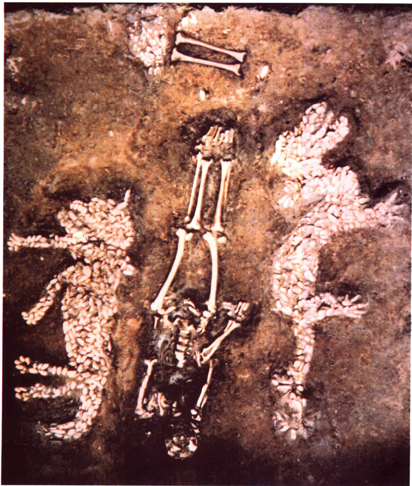
彩图版 1 河南省濮阳县出土的龙虎北斗图(约 6 千年前)
