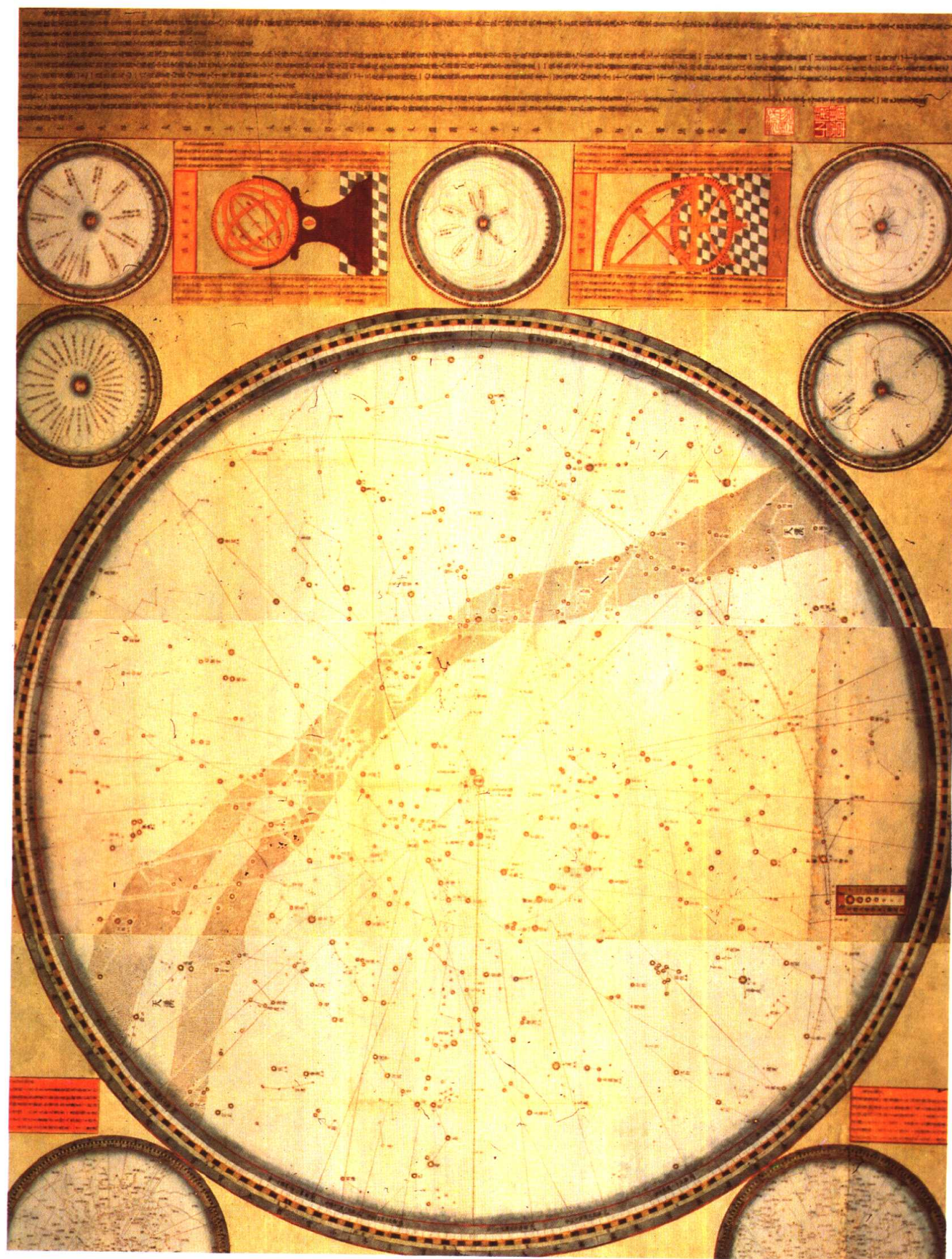
彩图版 10—1 《赤道南北两总星图》(赤道北星图),系由四幅屏风拼成(徐光启等 1634 年绘),现藏中国第一历史档案馆,由比利时鲁汶大学南怀仁中心提供
