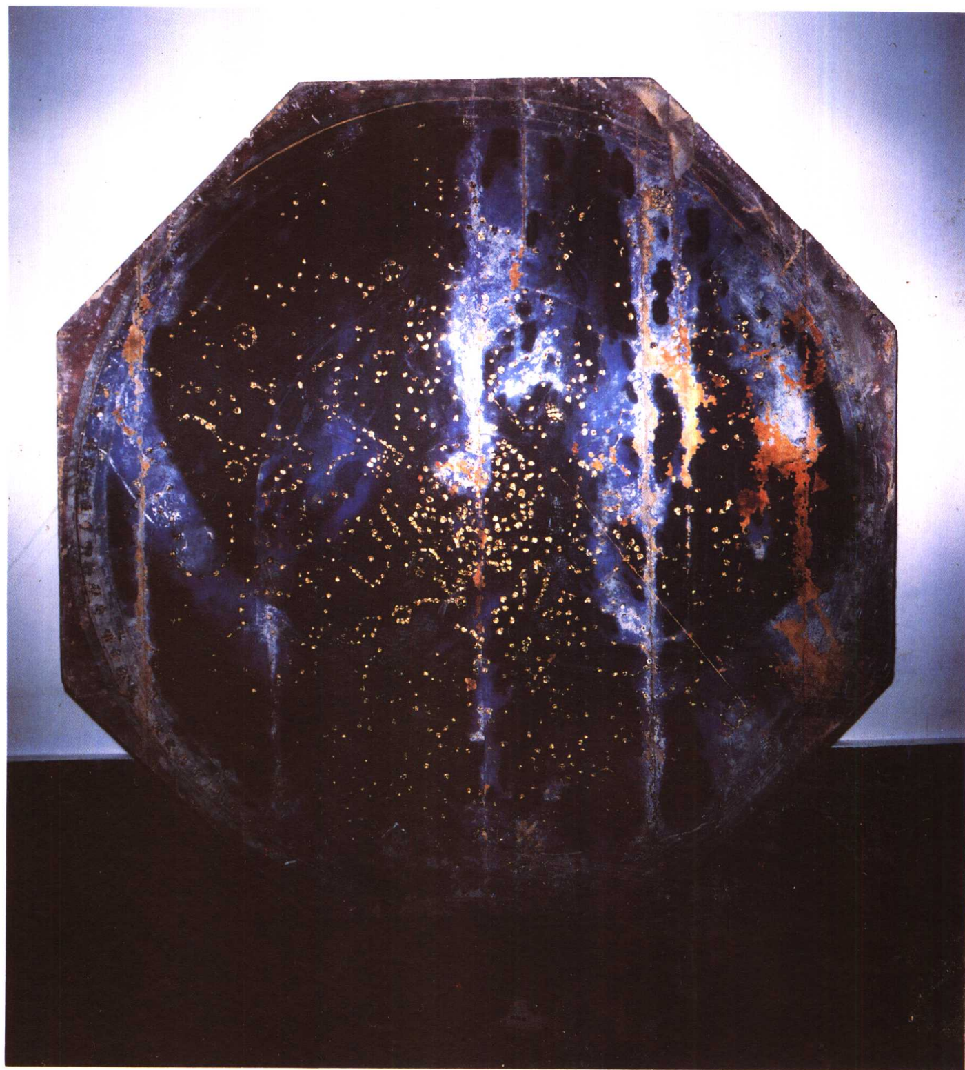
彩图版 7—1 北京隆福寺正觉殿藻井星图(约 1453 年)原图,伊世同提供
