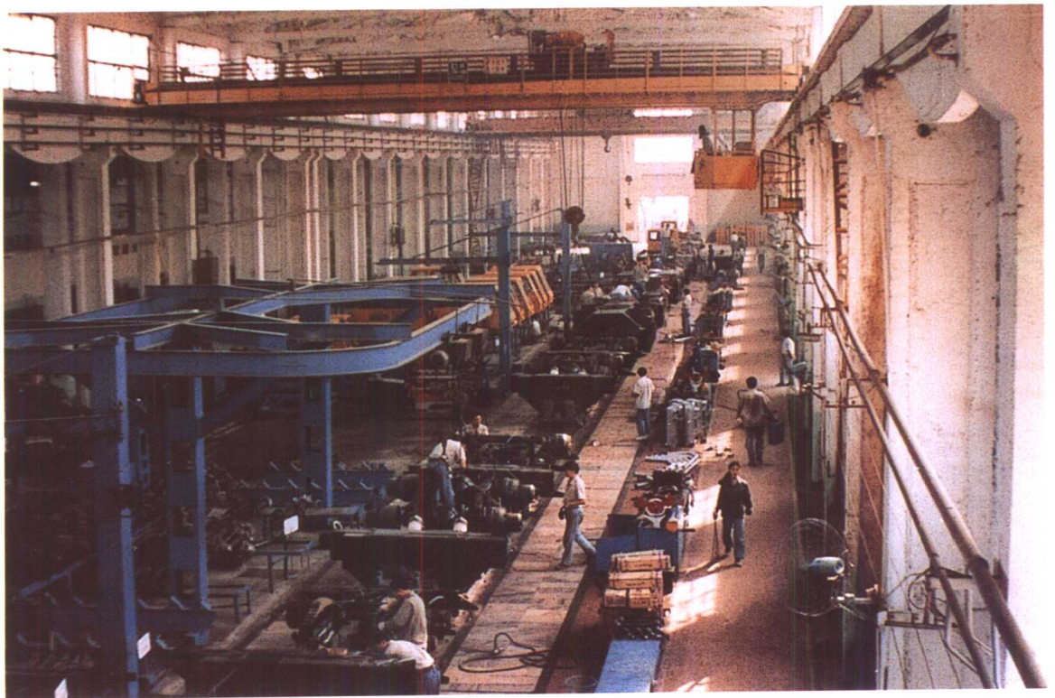
△ 徐州工程机械厂工程机械专用底盘生产线
