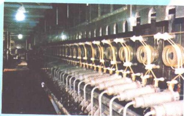
成都化学纤维厂粘胶短纤维纺丝机(1985 年)
