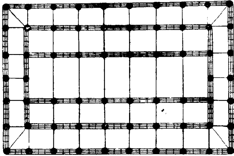
殿閣地盤殿身七間副階 周市各兩架椽身內雙槽
