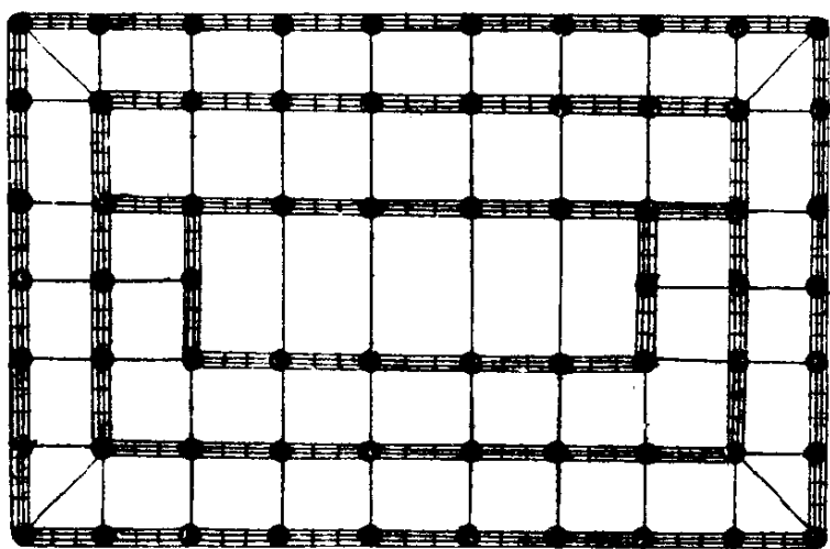
殿閣地盤殿身七間副階周市 各兩架椽身內金箱斗底槽
