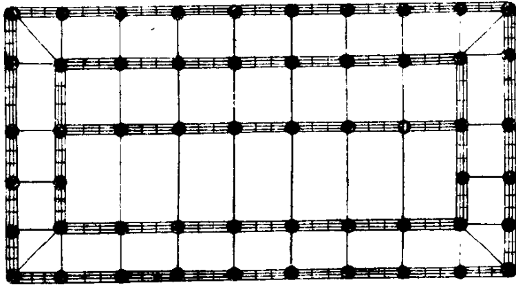
殿閣地盤殿身七間副階 周市各兩架椽身內單槽
