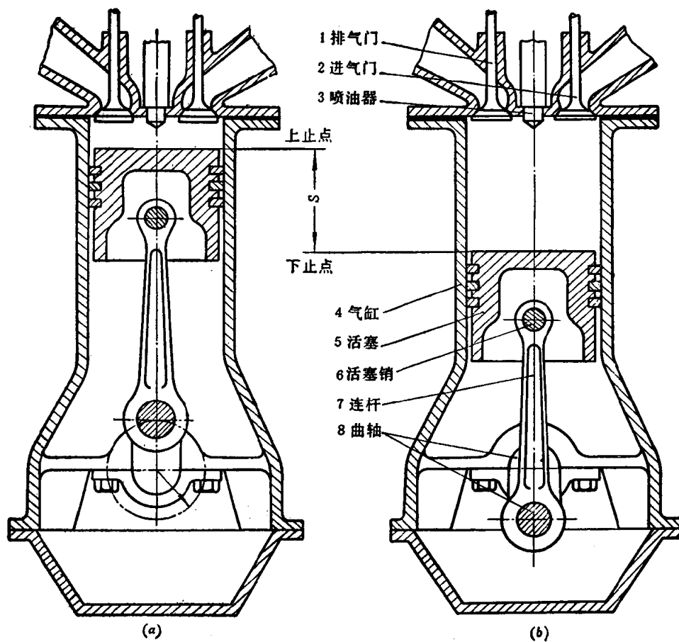
图1-1 单缸四行程柴油机简图
