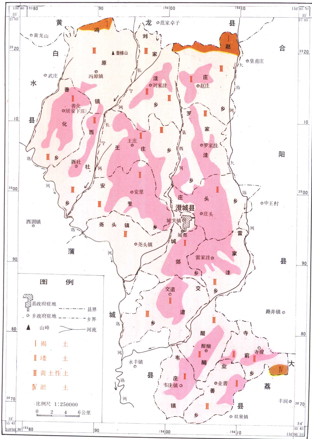
澄城县土壤分布示意图
