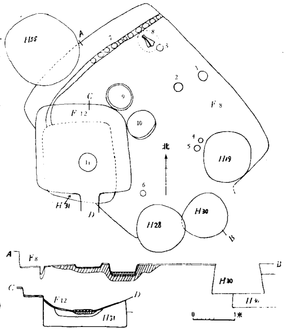
图七 F8、F12 平、剖面图
