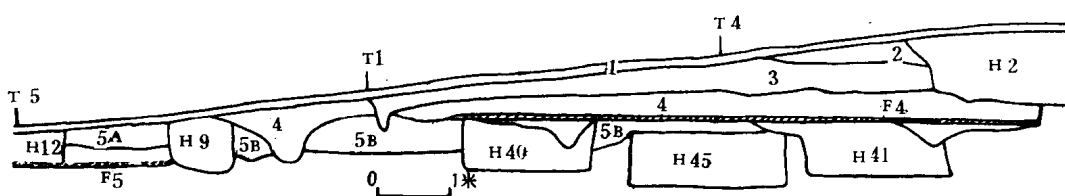
图二 BXT4、1、5西剖面图
