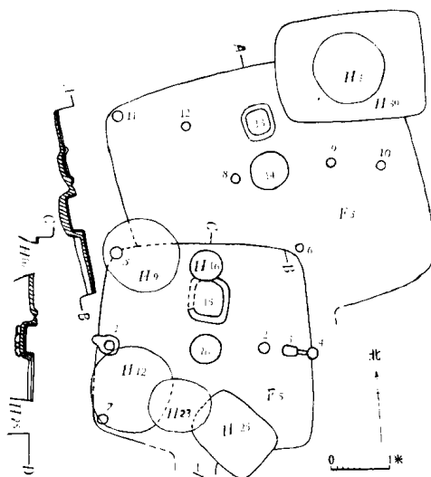
图四 BXF3、5 平、剖面图
