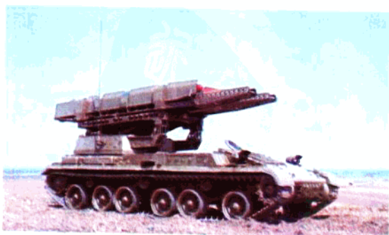
425 mm 火箭扫雷系统
