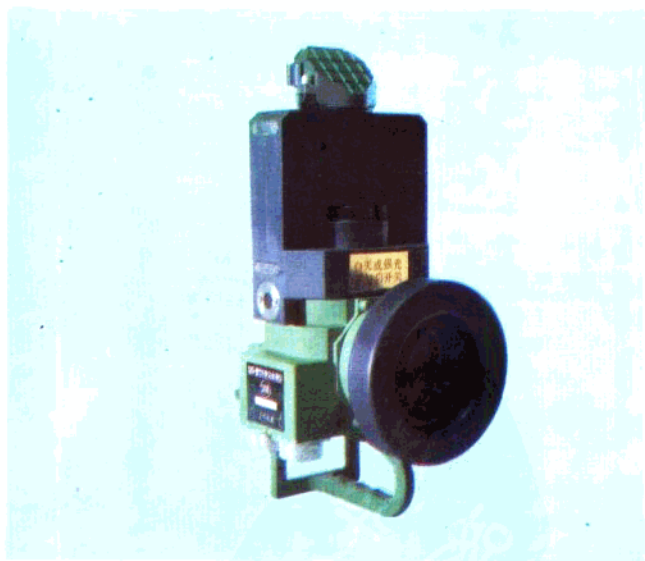
TDPN-2 型坦克驾驶员用夜间观察镜
