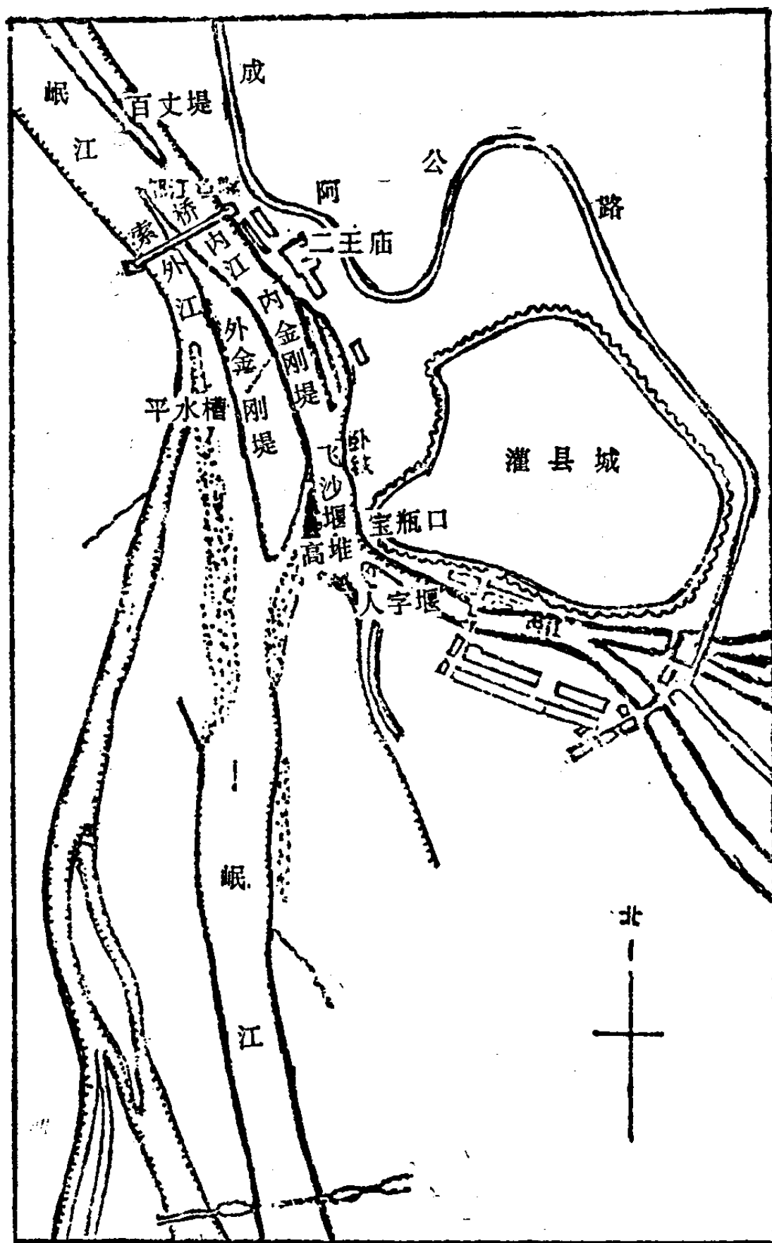
都江堰简图
