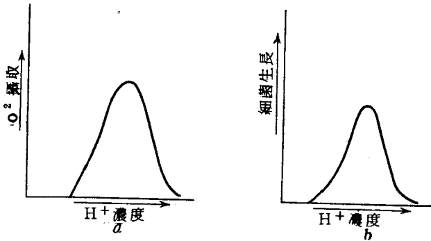
圖 1.3 氫離子濃度對 (a) 組織對氧的利用及 (b) 細菌的生長率之影響。
