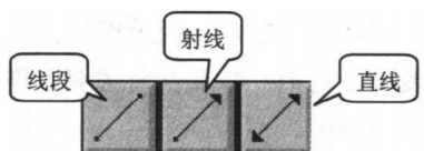
图 1.6 “画线”工具
