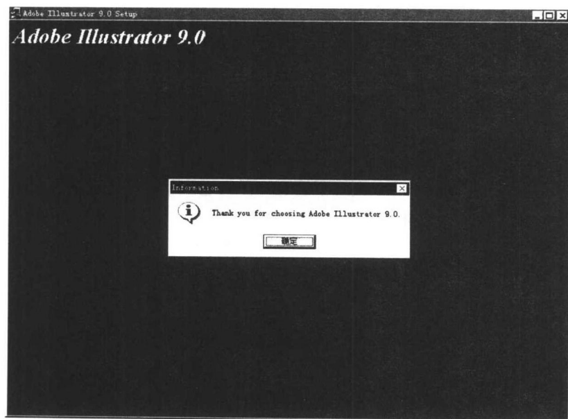
图 1-12 Information 对话框
