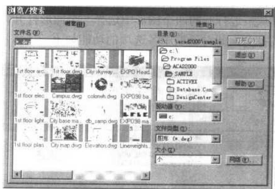
图 1-7 “浏览”选项卡
