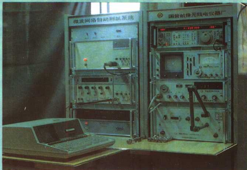
①⑦微波网络自动 测试系统
