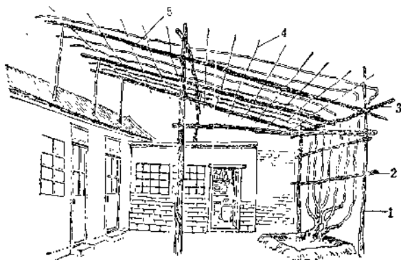
图 1 1.立柱 2.平杆 3.椽 4.竹椽 5. 梁 架长约 500 厘米，宽约 360 厘米，根部高约 320 厘米， 端部高 500 厘米，竹椽间距 45 厘米
