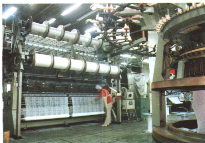
太仓针织总厂 经编双针床生产流 水线
