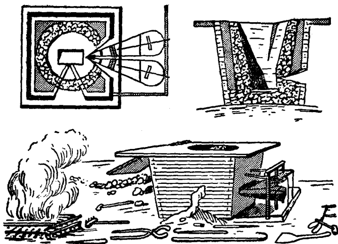
圖一 歐洲中世紀冶煉出熟鐵塊的冶鐵爐
