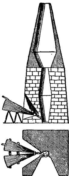
圖三 歐洲十八世紀初期的冶鉄鼓風爐
