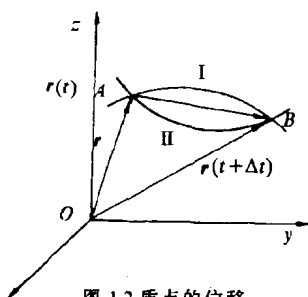
图 1-3 质点的位移
