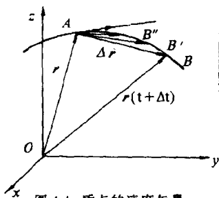
图 1-4 质点的速度矢量
