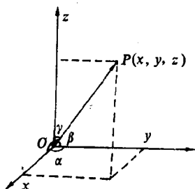
图 1-2 质点的位置
