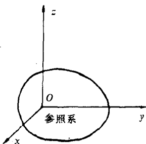
图 1-1 直角坐标系示意图
