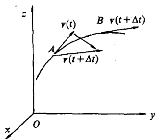
图 1-5 质点加速度矢量
