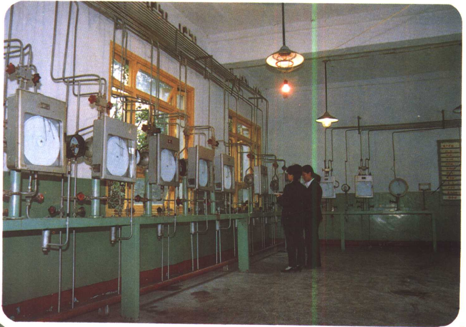
天然气配气站仪表间
