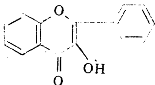
黃鹼醇 (flavonol)
