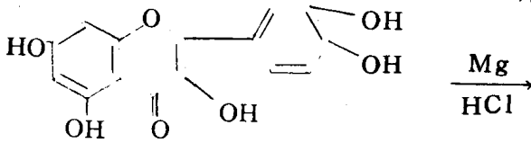
槲精 (Quercetin)
