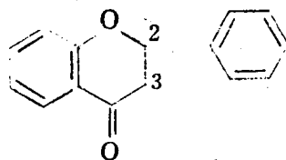
黃鹼酮 (flavonone)
