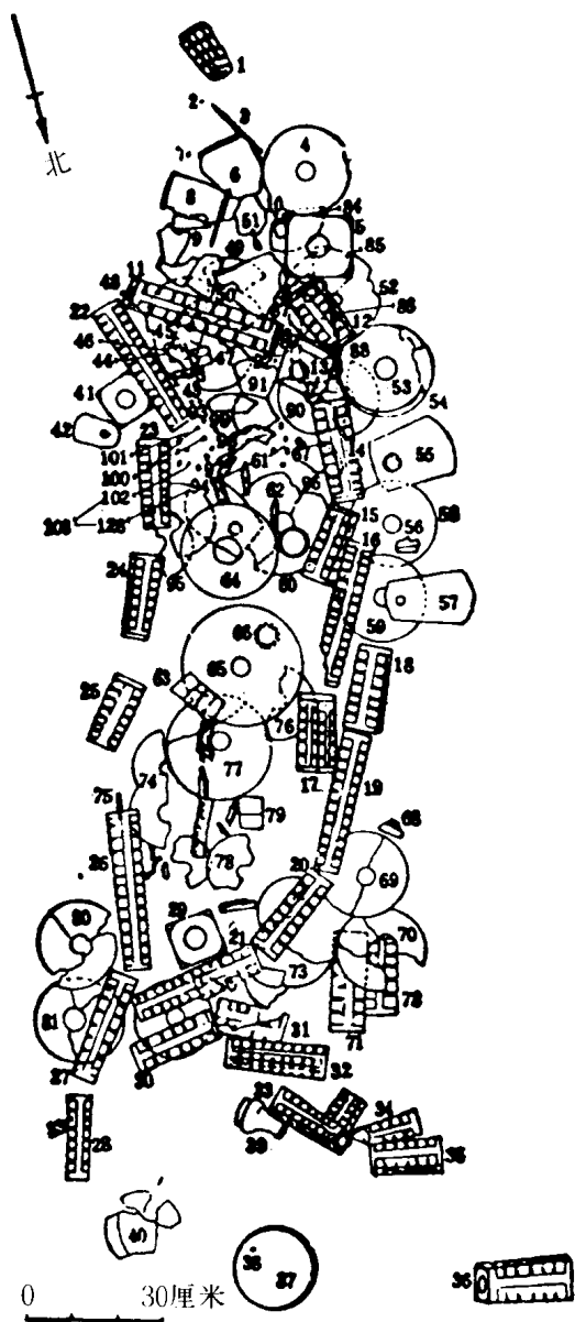
圖十四 寺墩3號墓平面圖
