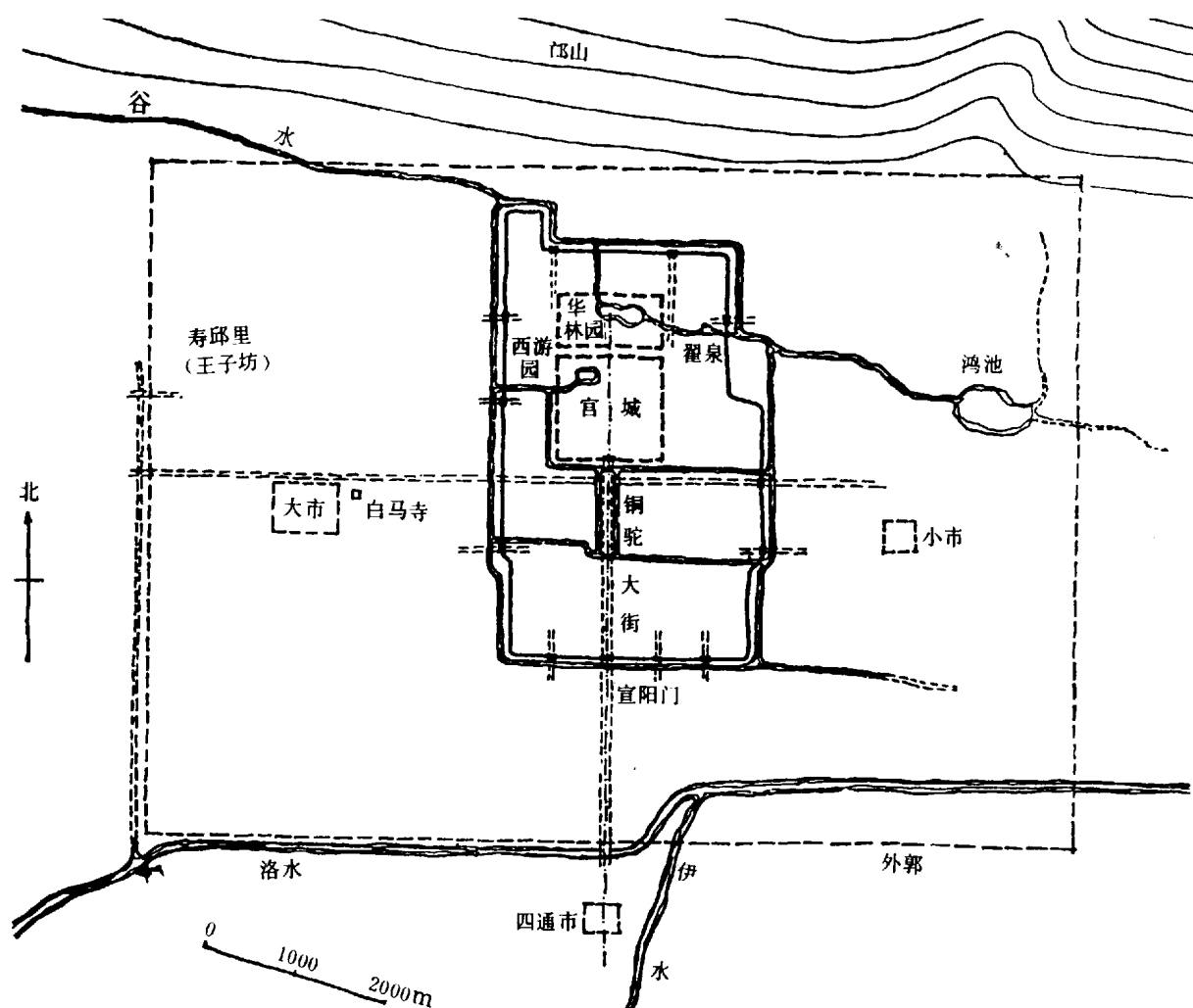
图 1—1 北魏 洛阳 主要官苑分布示意图 （引自清华大学《建 筑史论文集》六）
