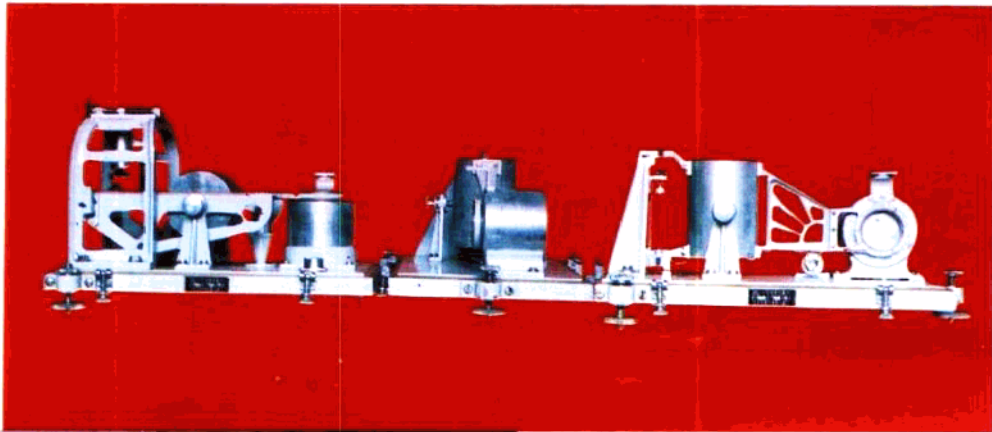
地震仪（左为垂直向，中、右为水平向）
