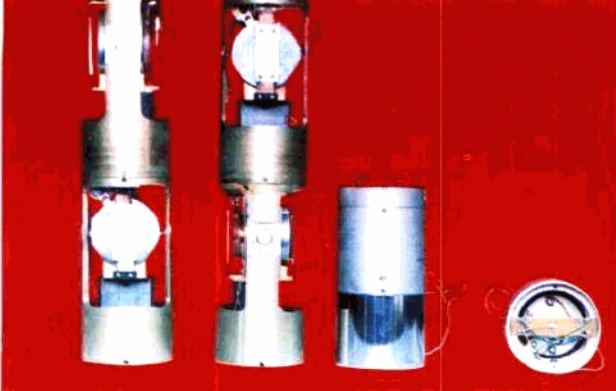
井下测震仪（左为水平向、右为垂直向）
