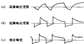
图 2.2 传输对脉冲信号的影响
