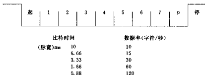
图2.6 起止式字符与传送时间的关系
