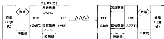
图 1.1 数据通信系统框图
