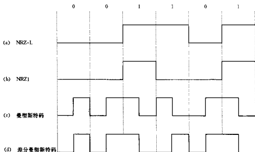
图 2.1 数字信号的编码
