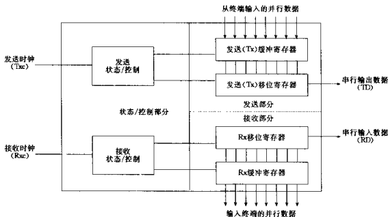
图 1.2 DTE 的简单示意图
