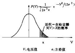
图 2.3 高斯分布
