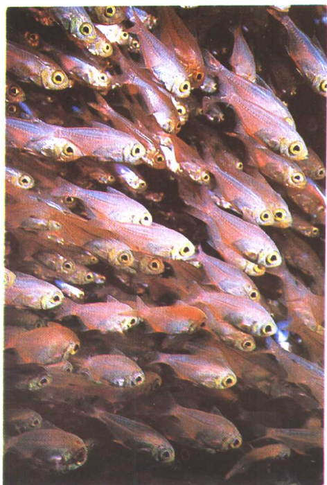
金眼鱼
