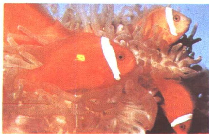
熊身鱼
