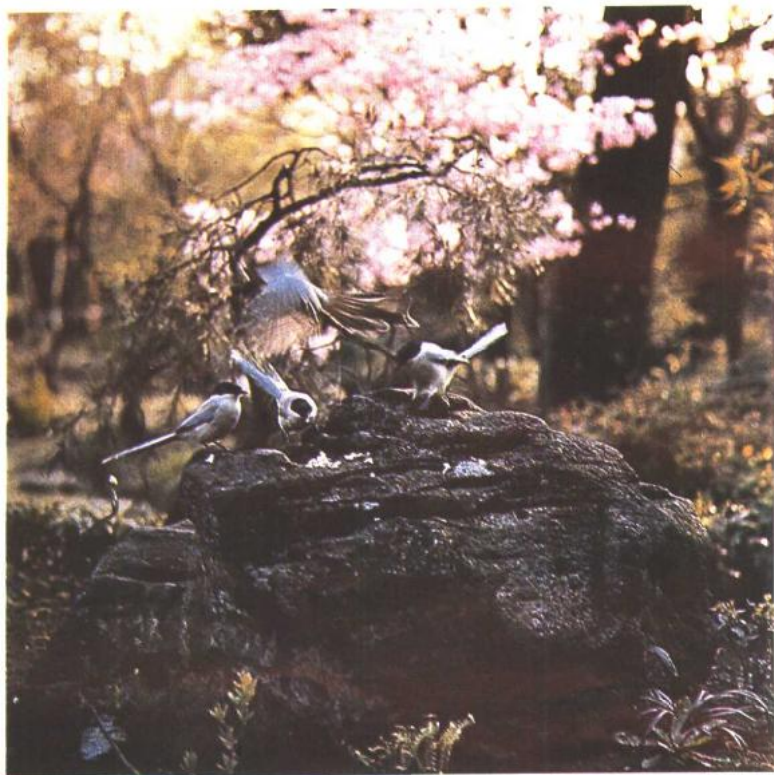
长尾鸟
