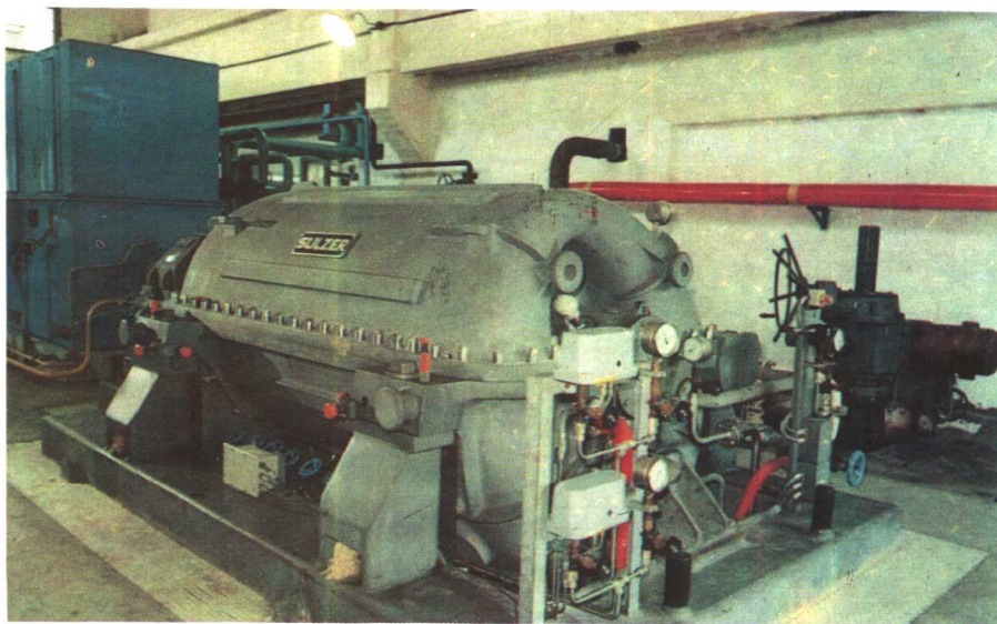
▽30万吨/年真空制盐生产装置及主控室
