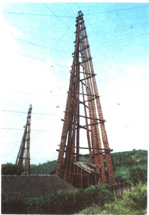
◁大14井、新大6井天车(两井分别高80余米)
