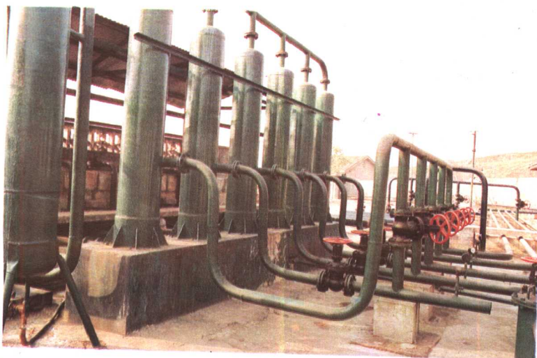
△卤井压裂
