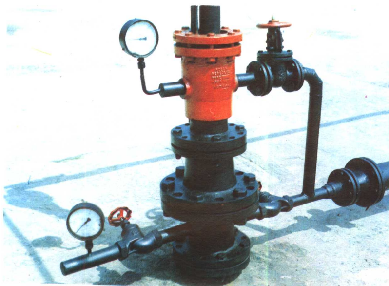
▽潜卤泵采卤
