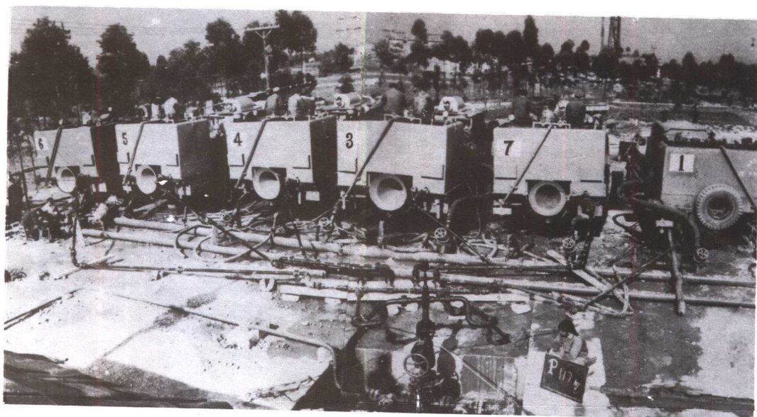
△卤井压裂
