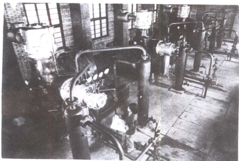
△气举采卤
