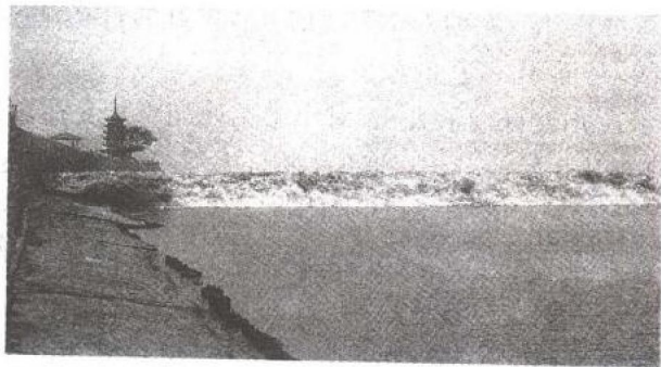
钱江大潮
