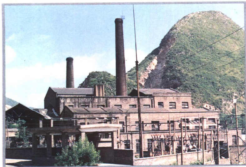
县火电厂
