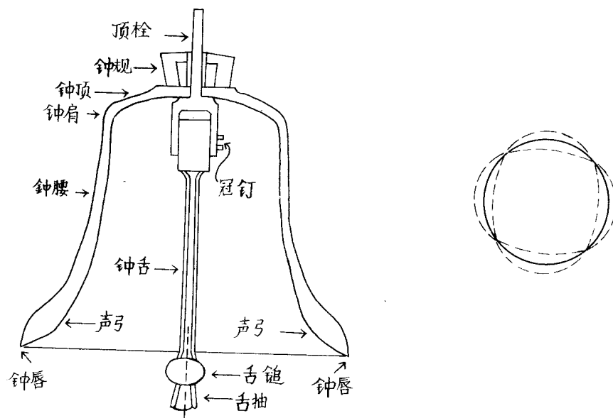
图二十八 欧洲圆钟及其四节线周向振动示意图
