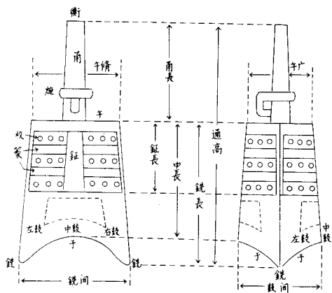
甲、编钟各部分名称、位置及其大小示意图
