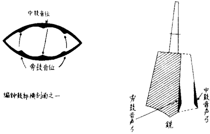
乙、编钟横剖面及纵剖面例示
