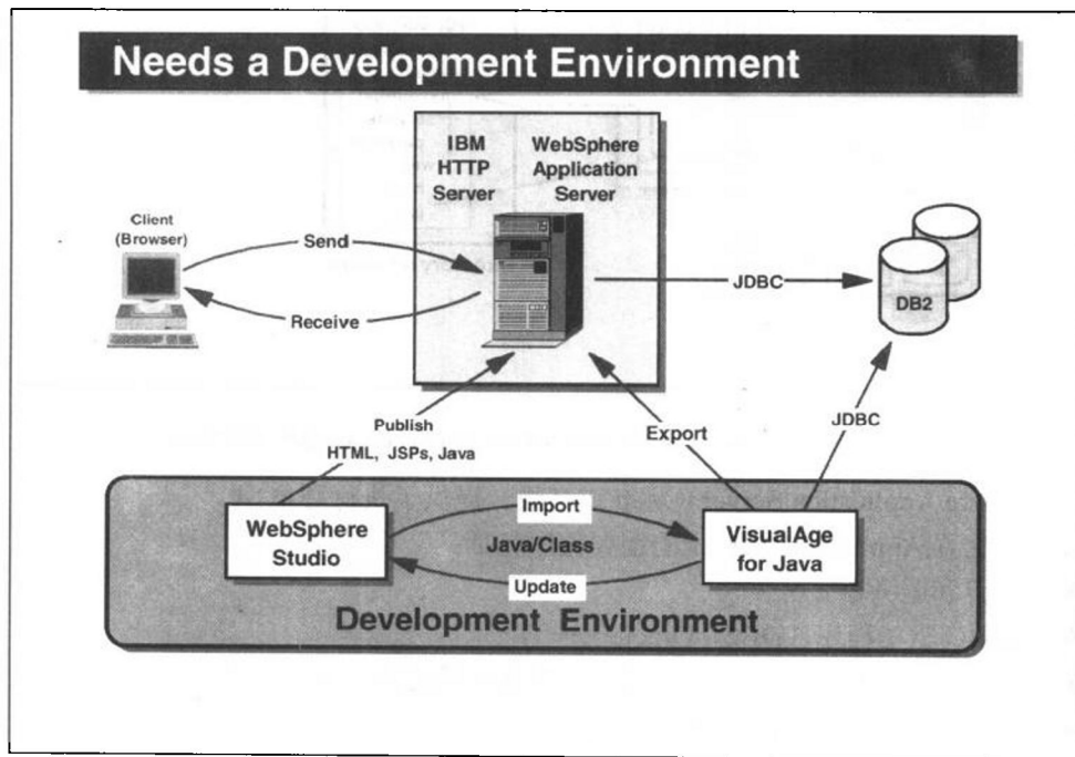
图 1-9 需要一个开发环境
