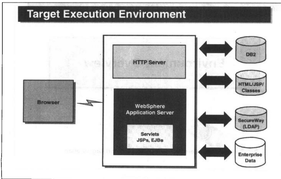
图 1-8 目标运行环境
