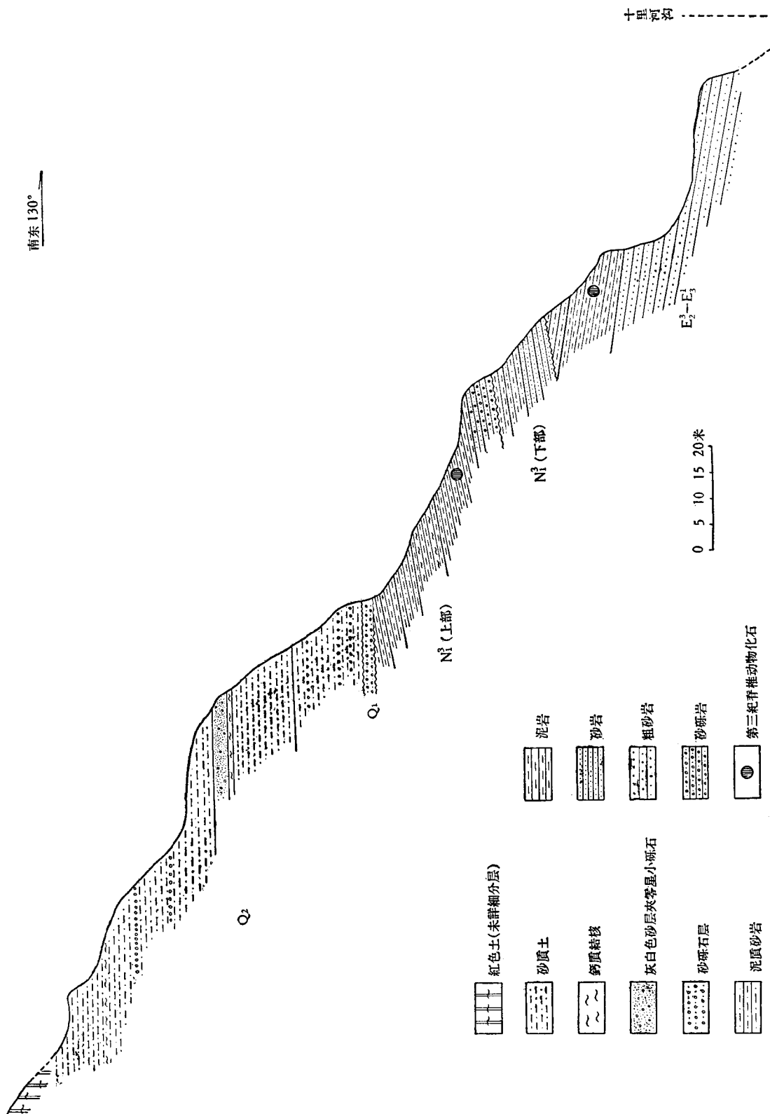
图 3. 高坡村北上中新统寇家村组剖面图
