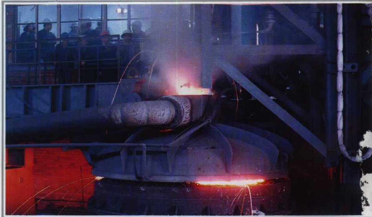
● 攀钢以质量求信誉，从联邦德国引进了TN喷粉装置，保证了钢的质量
