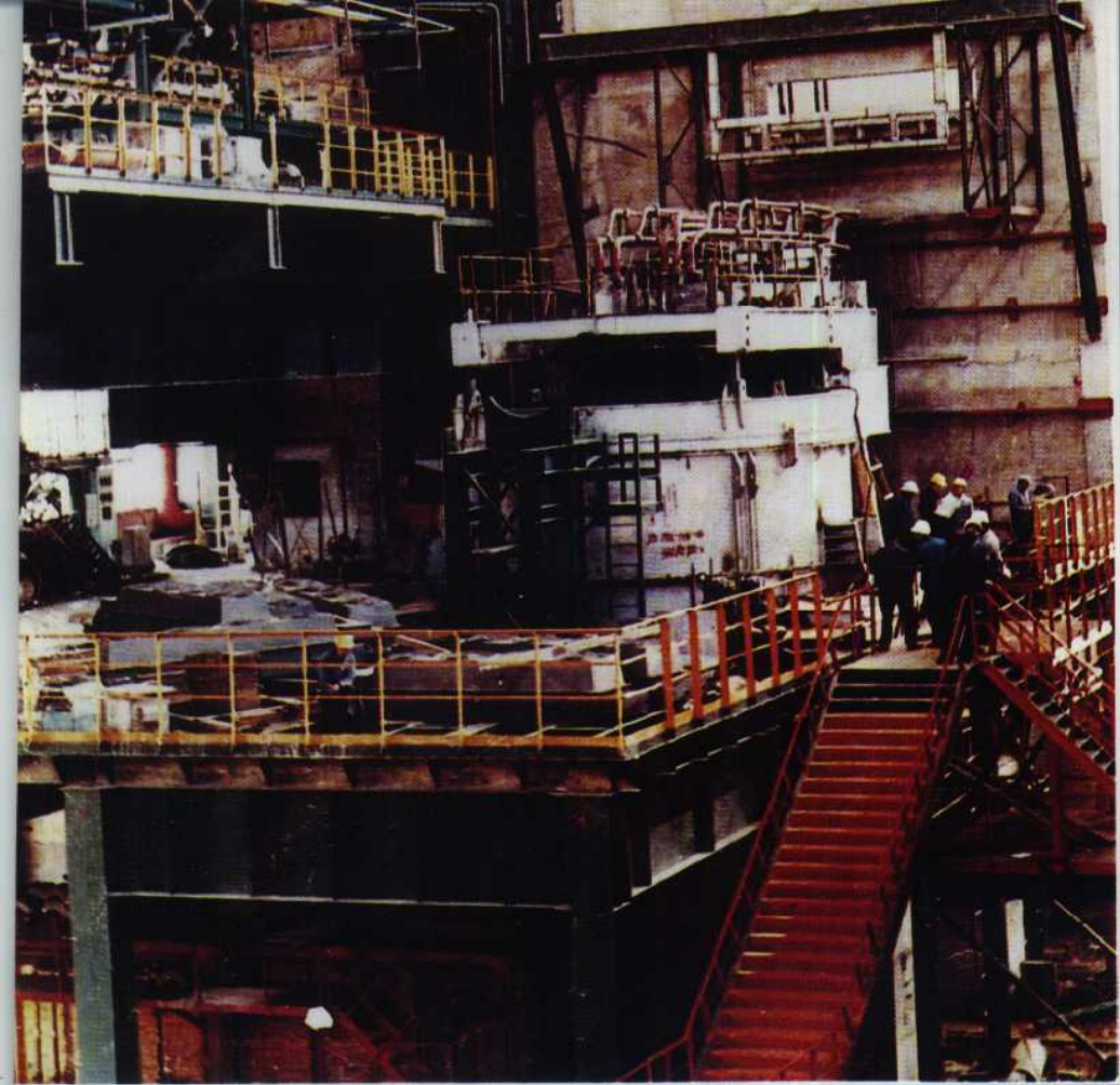
● 75吨电弧炉正在舞钢安装
