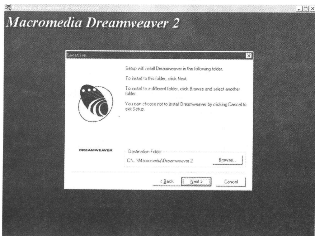
图 1.4 Location 对话框
