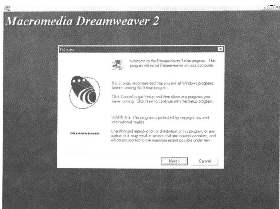
图 1.3 Welcome 对话框
