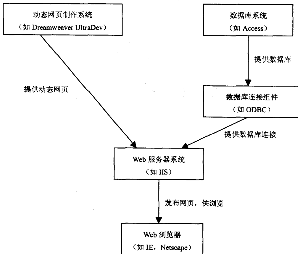
图1.1 Web开发系统
