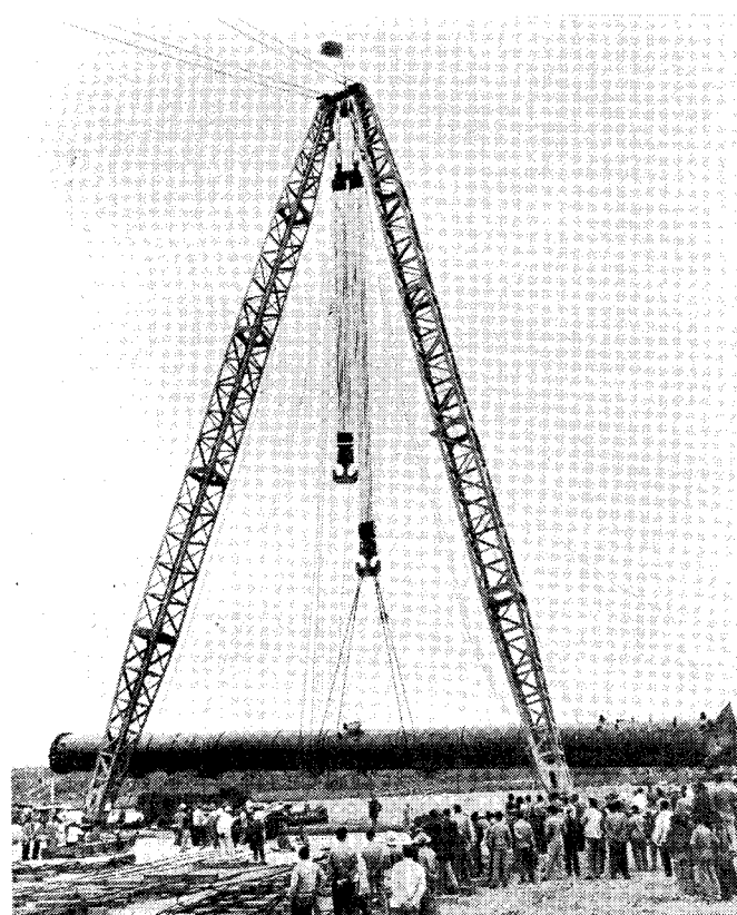
我国第一座大型外海岛式码头——陈山原油码头胜利建成
