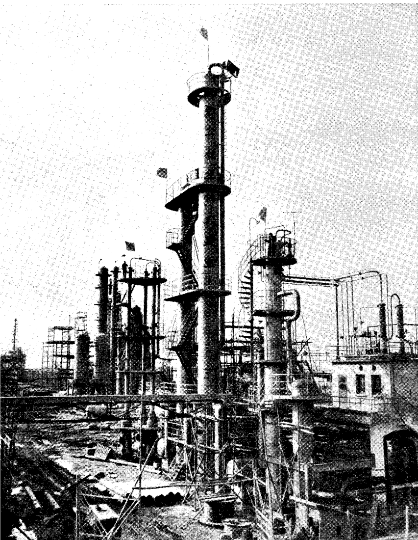
我国自行设计、自行制造的“外冷却”醋酸装置全貌
