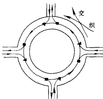
图 1.2.6 相交冲突点的分散 (三)转盘式
