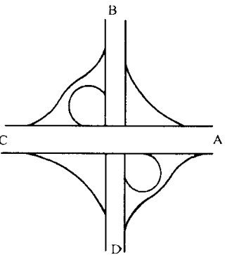
图 1.4.3 例 1.4.1 中的立交设计图式
