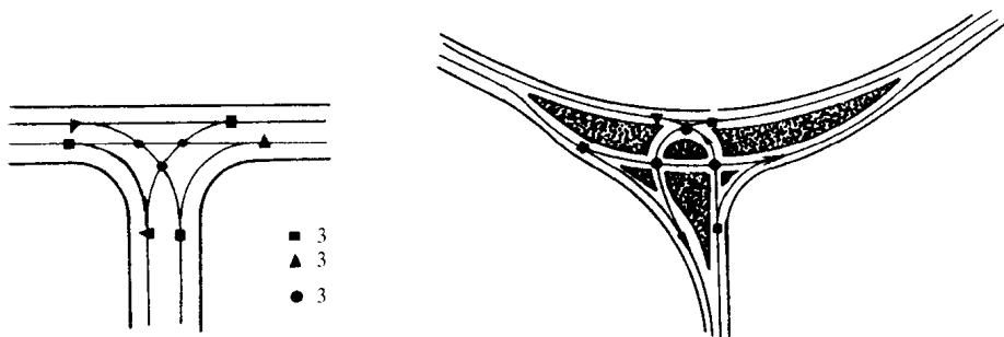
图 1.2.10 相交冲突点的分散 (七)T 形交叉,车道分开
