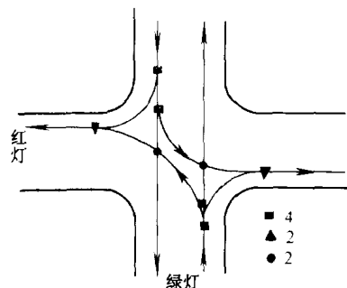
图 1.2.7 相交冲突点的分散 (四)红绿灯控制
