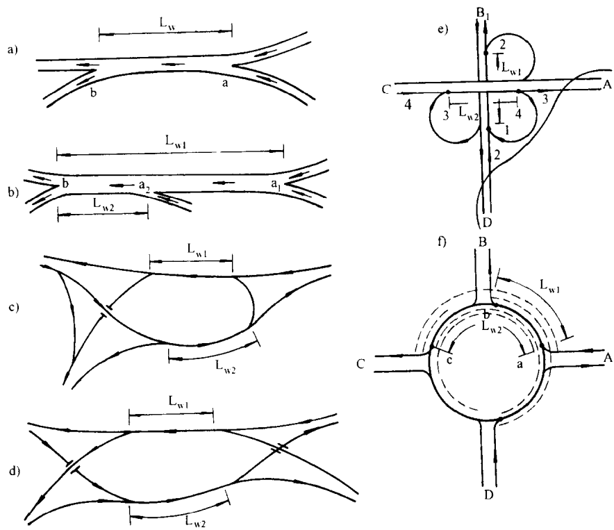
图 1.5.1 交织段的各种情况
