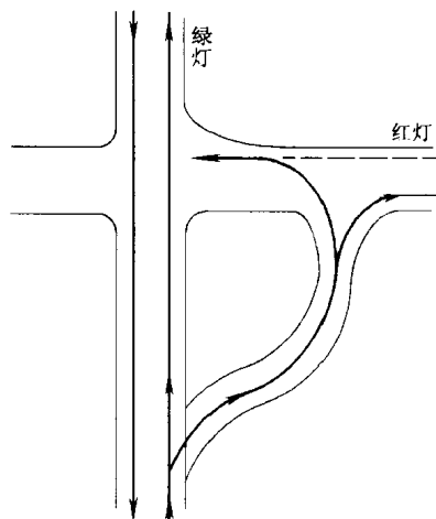
图 1.2.9 相交冲突点的分散 (六)壶把式交叉
