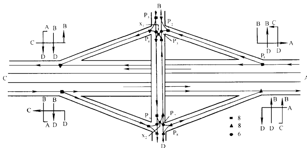
图 1.4.1 菱形互通式立交的冲突点(一)
