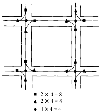
图 1.2.5 相交冲突点的空间分散 (二)两条道路的上、下行车道都分开
