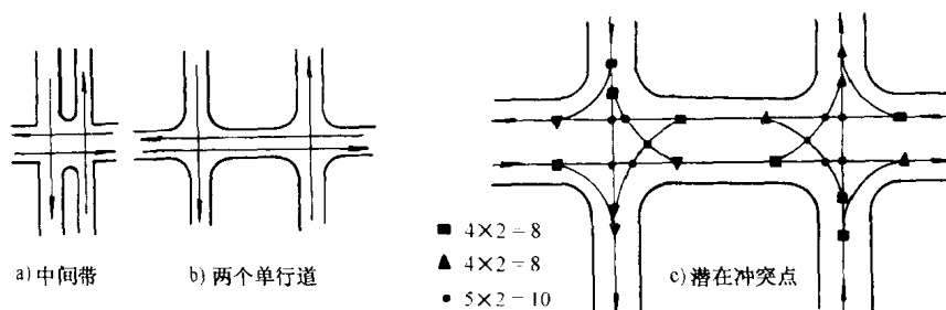
图 1.2.4 相交冲突点的空间分散
