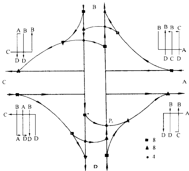
图 1.4.2 菱形互通式立交的冲突点(二)
