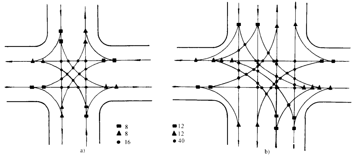
图 1.2.3 十字交叉路口的潜在冲突点
