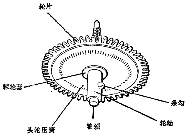
图 1-5 走头轮组件 (背面)
