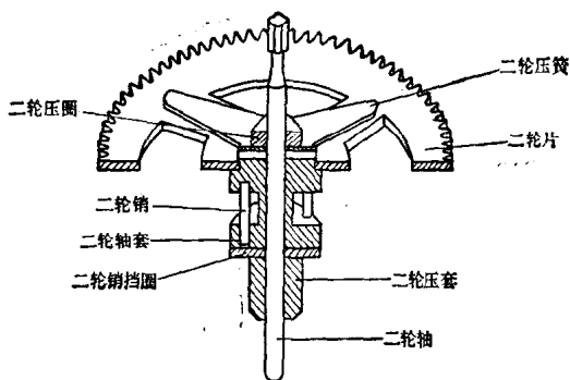
图 1-6 二轮组件剖面图
