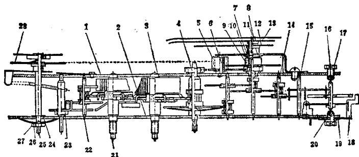
图 1-3 机心展开图
