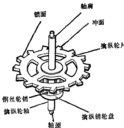
图 1-8 擒纵轮组件
