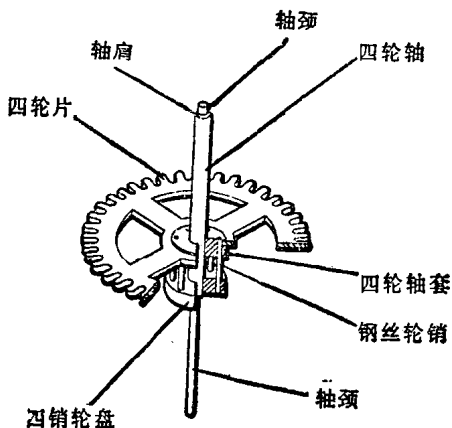
图 1-7 四轮组件剖面图
