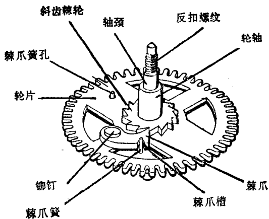
图 1-4 走头轮组件 (正面)
