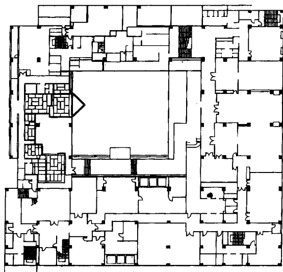
三层平面图
