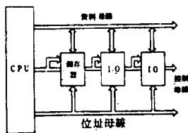
位址母線
