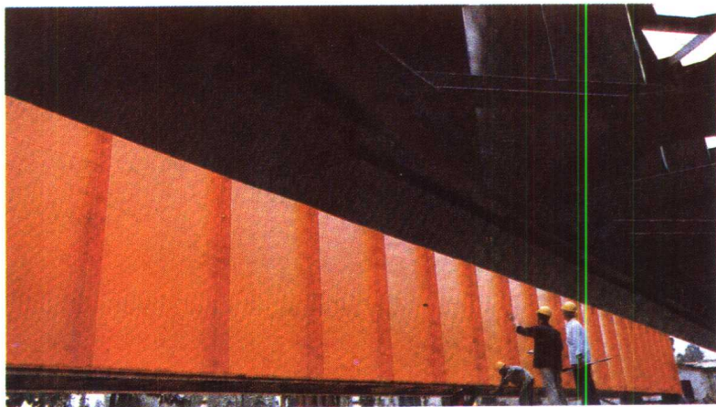
山海关桥梁厂生产的 黄河大桥桥梁
